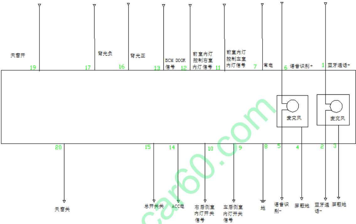
后室内灯
