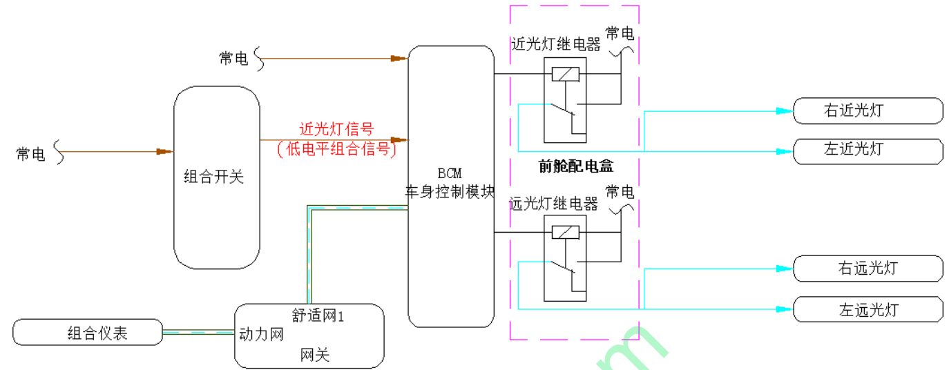
系统框图
