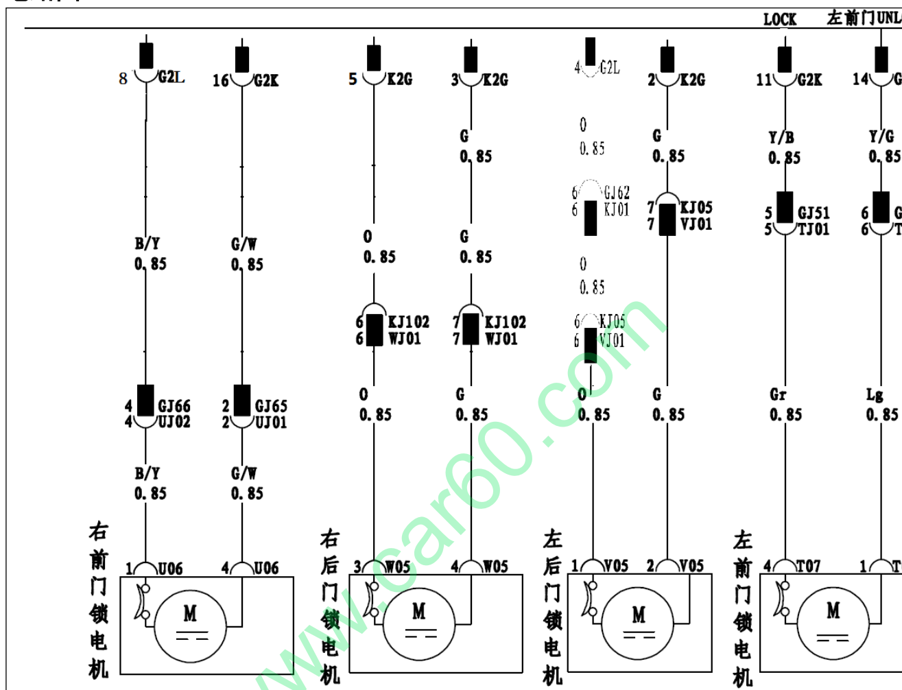
电路图
